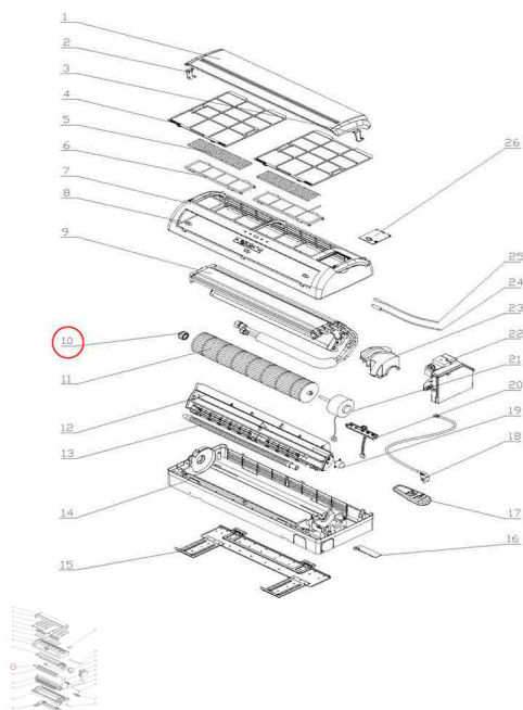
Rodamiento + soporte para eje de turbina Airwell (4523526)
