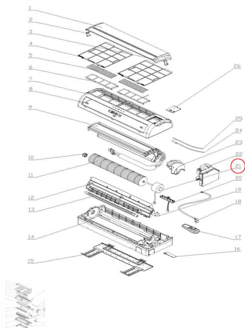
Motor ventilador DIE 20-30 WDI 9-12 MAE (453088600)
