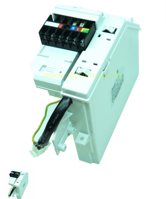
Conjunto electrónica MAE-45 AIRWELL JOHNSON (453101900R)
