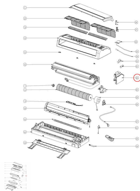
Conjunto electrónica DIE 45 WDI 18 Johnson Airwell 467300006R
